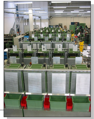
Ansicht: Pressen 3
